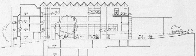
Schnitt Studios-Zugangsrampe 1:750
