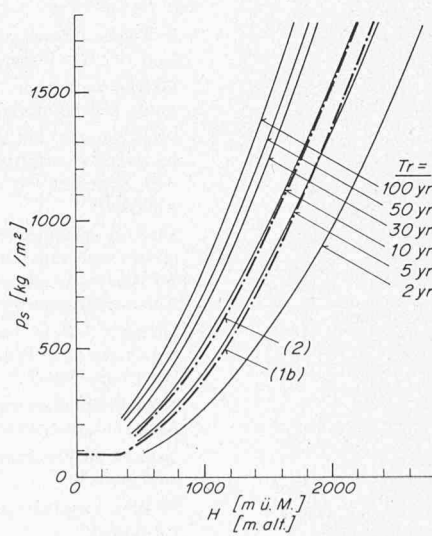
Bild 2. Gemessene, aber durch Ansätze ausgeglichene Extremwerte der Schneelasten p_s als Funktion der Meereshöhe für die Wiederkehrsdauer T_r = 2 Jahre, 5 Jahre, 10 Jahre, 30 Jahre, 50 Jahre und 100 Jahre. Strichpunktiert sind auch die Werte nach Gl. (1b) und (2) eingetragen
