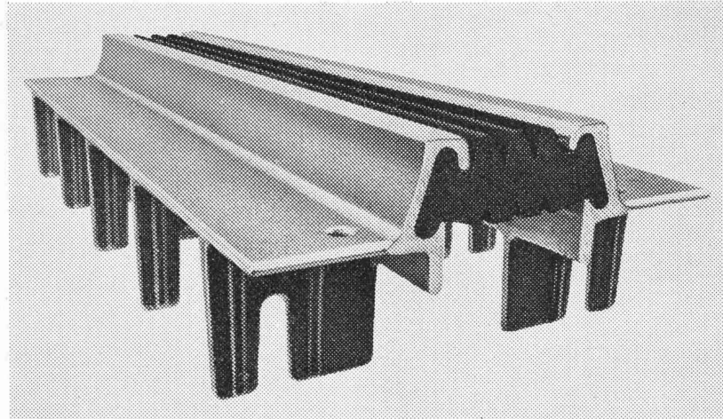
RIPPENFUGE — eine starr einbetonierte robuste Fahrstufe aus feuerverzinktem Kugelgraphitguss.
