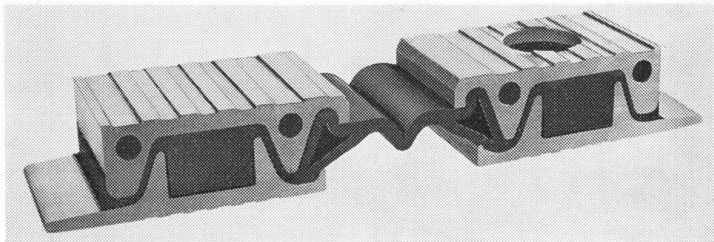
ELASTFUGE — eine vorgespannt verankerte, hochelastische Fahrstufe aus Aluminium-Neopren Verbundelementen.
