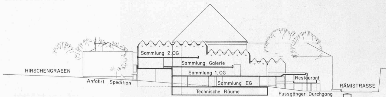
Schnitt Hirschengraben/Rämistrasse 1:900
