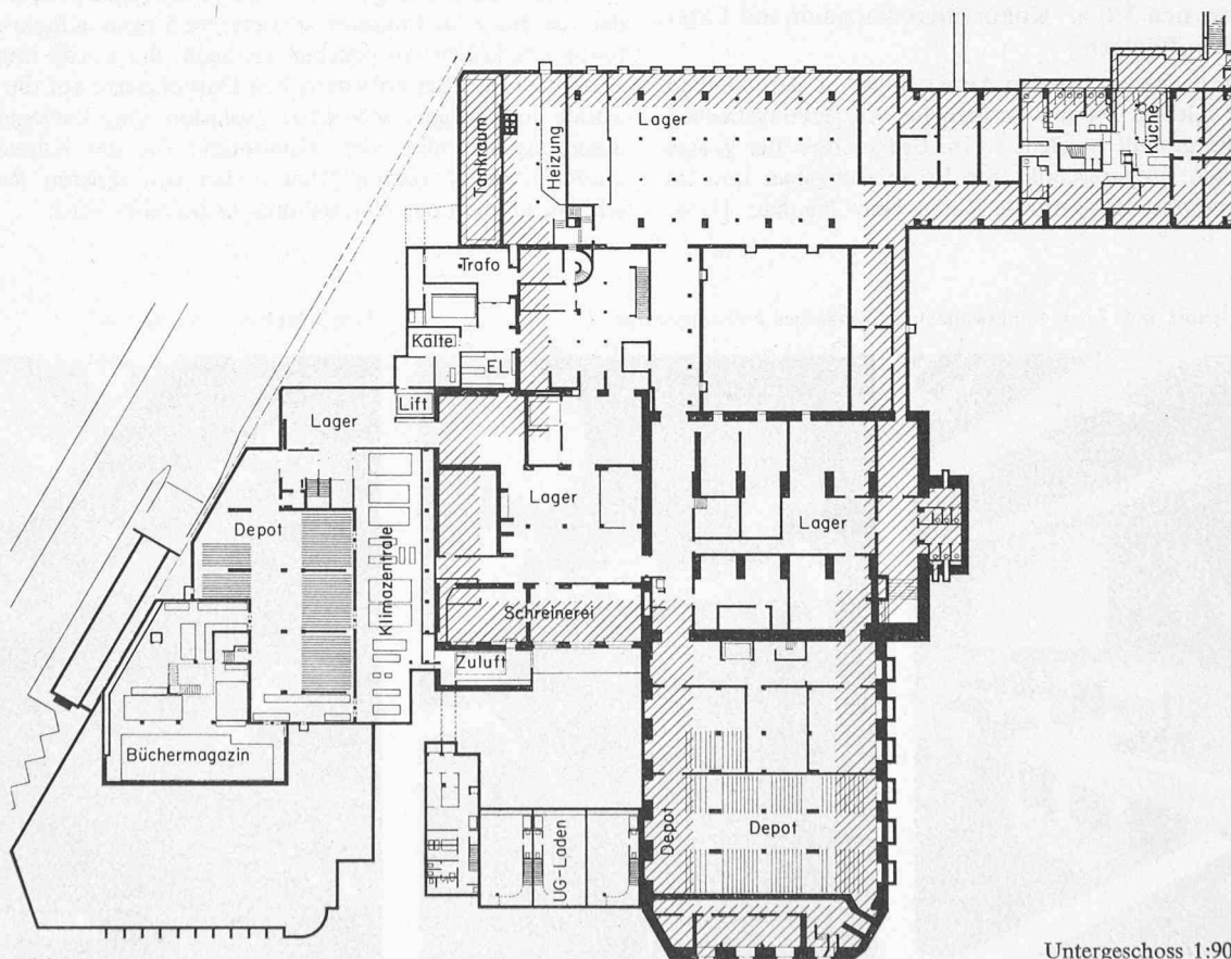
Untergeschoss 1:900
