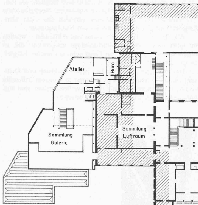
Galerie-Geschoss 1:900
