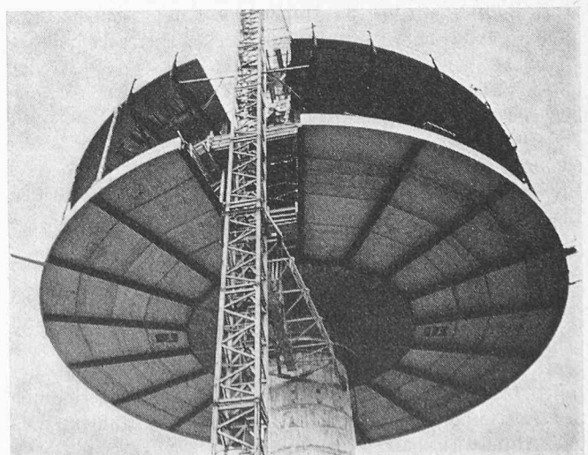
Bild 4. Kegelschale aus 48 Stahlbetonfertigteilen für die Plattform des Fernmeldeturmes in Kiel (Bild 1)
