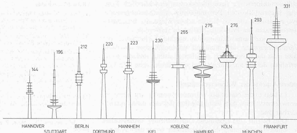
Bild 1. Einige Fernmeldetürme der Deutschen Bundespost in Sonderbauformen aus Stahlbeton
