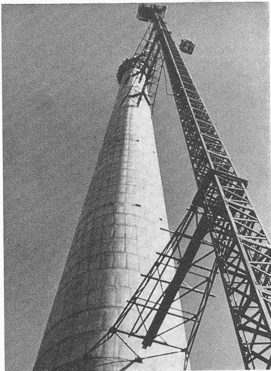
Bild 2 (links). Fernmeldeturm Koblenz (1974/75), beim Bau des Schaftes
