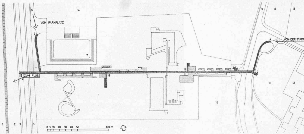
Situation (Strassengeschoss) von Schwimmbad und Kunsteisbahn Bellinzona (aus «WERK» Nr. 2/1971) Legende: 1 Markierung des linken Ticino-Ufers, 2/3 Uferpartie mit Spazierweg, 4 Zugang Passerelle (daneben Dienstgänge), 5 projektierte Autobahn (vgl. Flugaufnahme!), 6 Zugang vom Parkplatz, 7 Kunsteisbahn, 8 Parkplatz, 9 Umfahrungsstrasse, 11 öffentliche Parkanlage, 12 Kantonsschule, 13 Sportplätze, 14 Erweiterungsmöglichkeit, 15 Eingang für Schüler, 16 Haupteingang
