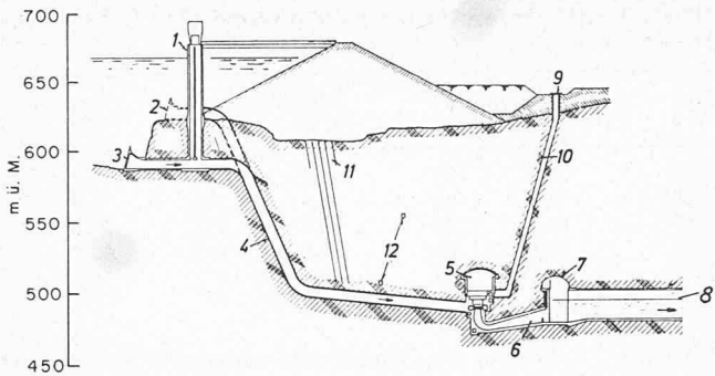
Bild 3. Längsschnitt der Kraftanlage G.M. Shrun. 1 Einlaufkontrolle, 2 und 3 Einlauf, 4 Druckrohre, 5 Maschinenhaus, 6 Auslass, 7 und 8 Ausgleichskammer und Ablass-tunnel, 9 Umspannstation, 10 Kabelschacht, 11 Abschrägung, 12 Entwässerungstunnel
