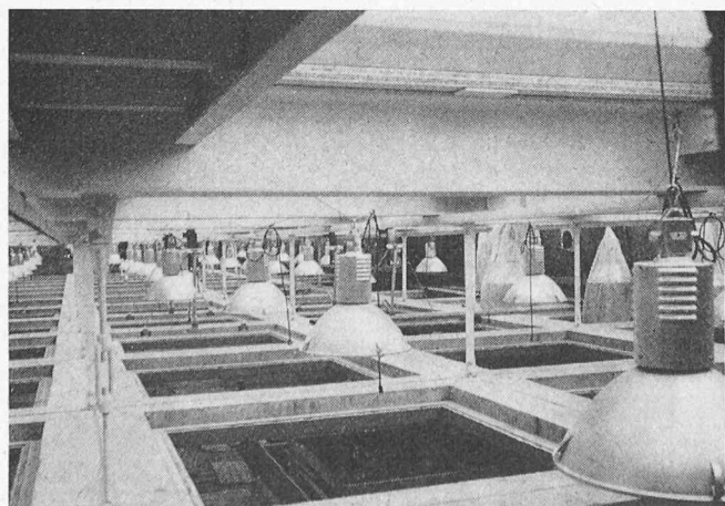
Überspannung des Lichthofes mit doppelschaligen Oberlichtkuppeln. Im Hohlraum sind Lampen angeordnet
