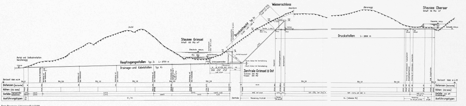
Erste Bauetappe, Längsprofil 1:2.500
