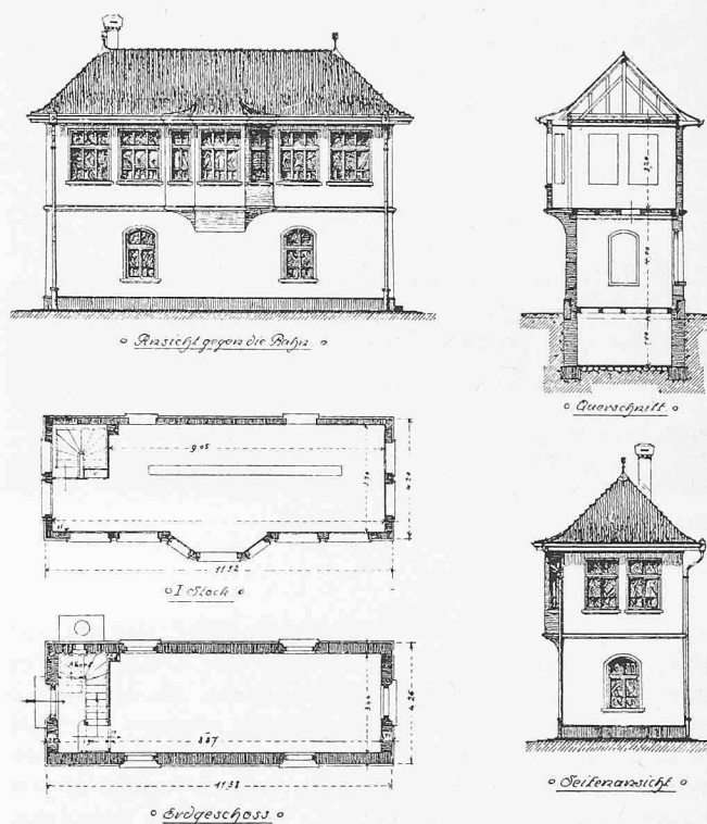
Stellwerkhäuschen
