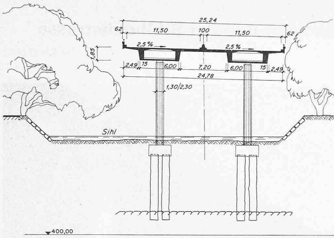
Bild 4. Querschnitt Pfeilerachse 125: Normalfeld
