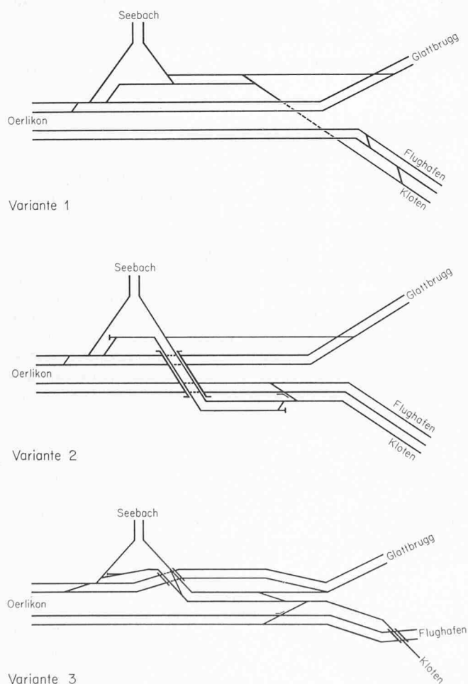
Bild 4. Systemskizzen für 3 verschiedene Lösungsmöglichkeiten der Verflechtungstrecke zwischen Oerlikon und Glattdrugg
