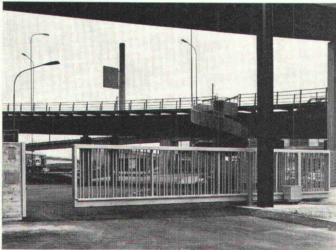
Beispiel eines freiaufragenden Arealtores mit Antrieb metoran
