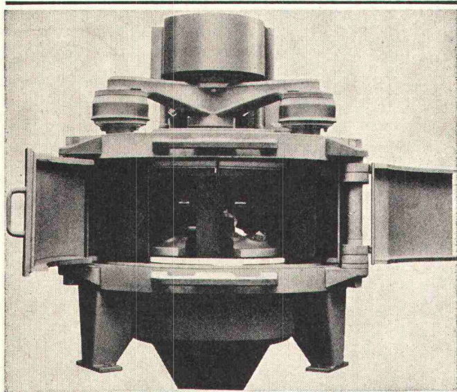
TURBO-Zentrifugal-Hammerbrecher Patent Pozzato
