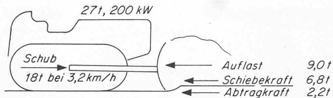
Bild 2. Hauptkräfte und Leistungen, die bei einer Planierdrape bei einem mit Vollast durchgeführten, 15 cm tiefen Schnitt auftreten
