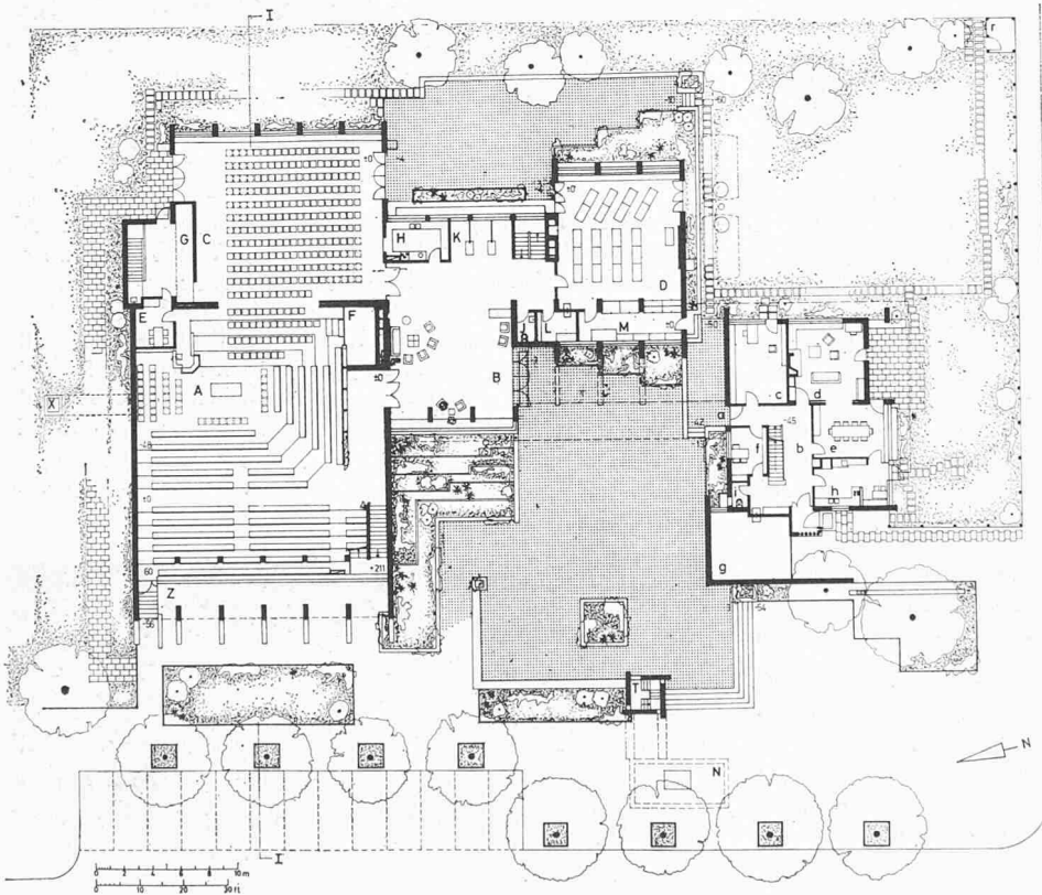
Hauptgeschoss 1:600
