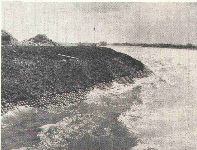
Bild 2. Ufersicherung am Kanal von de West (Niederlande)
