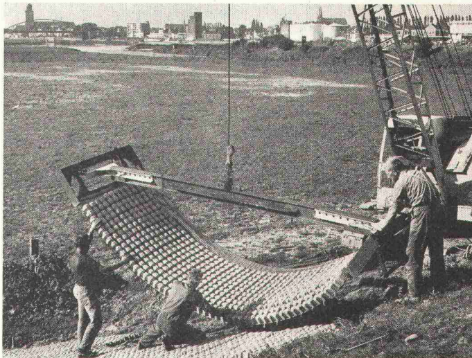
Bild 1. Verlegen von Gobi-Matten in Deventer (Niederlande)
