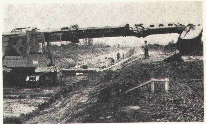
Bild 1. Aushub des Kanalprofils durch Teleskop-Bagger
