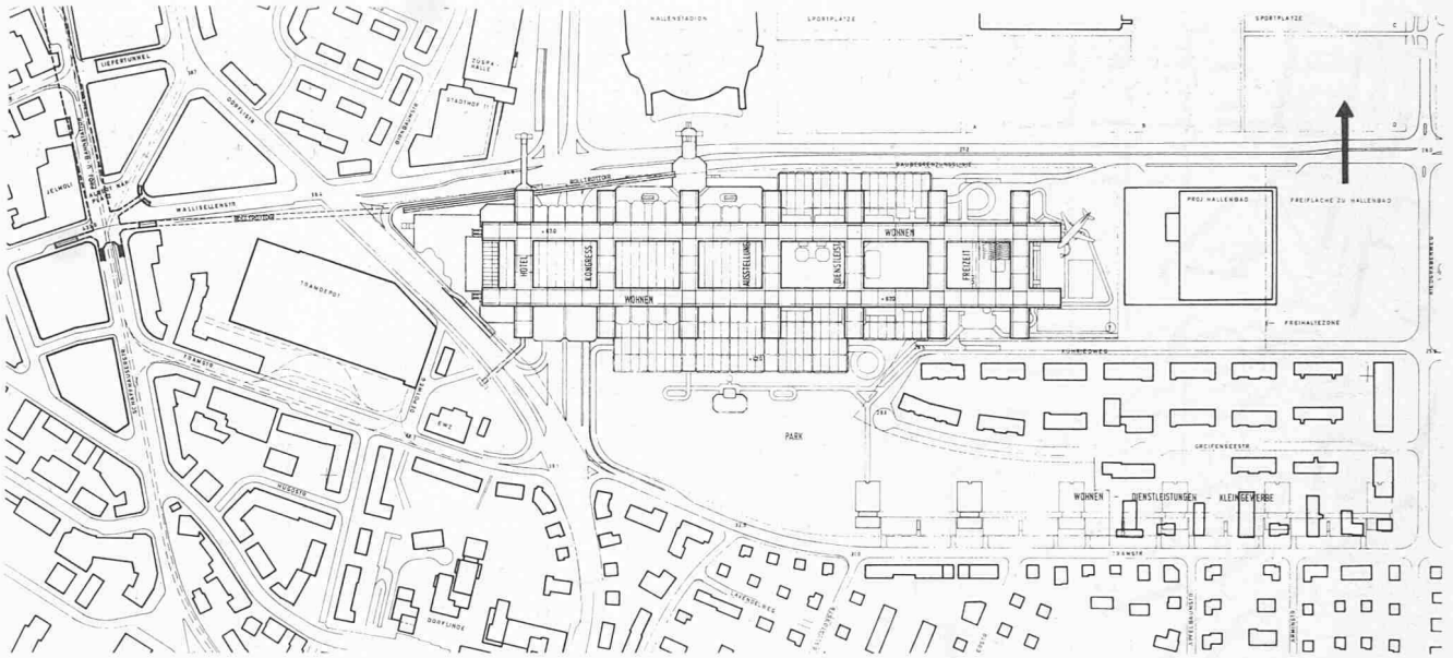
Situation 1:6000 zu Projekt 10. Preis
