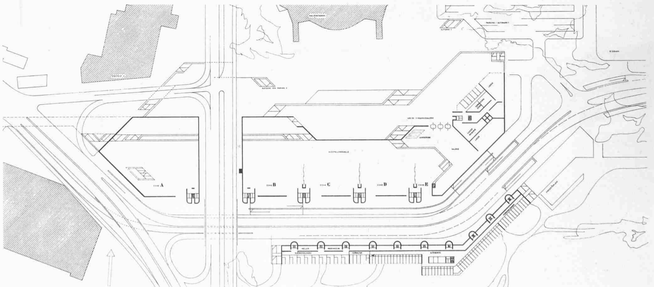
Geschoss 2, 1:3000 (Erdgeschoss)
