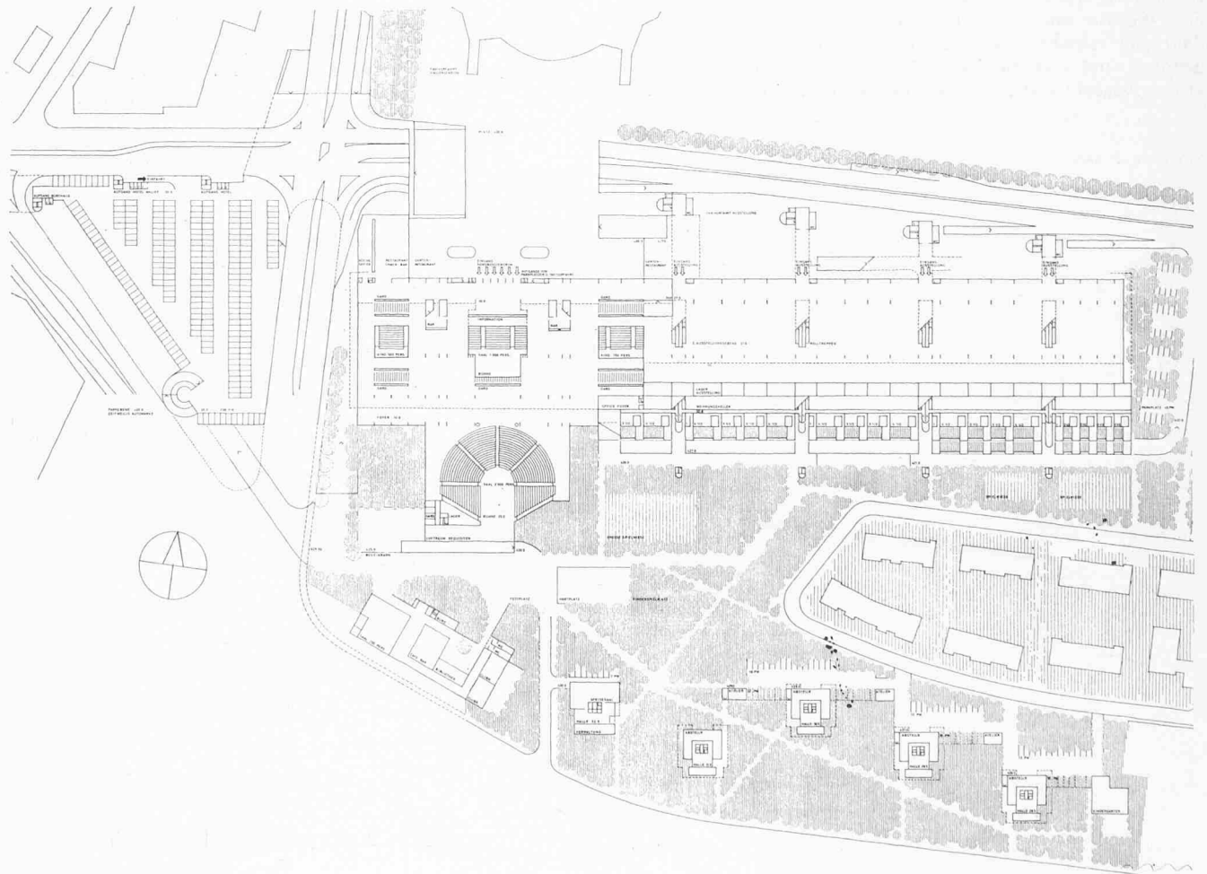
Grundrissebene 3, 1:3000, Erdgeschoss
