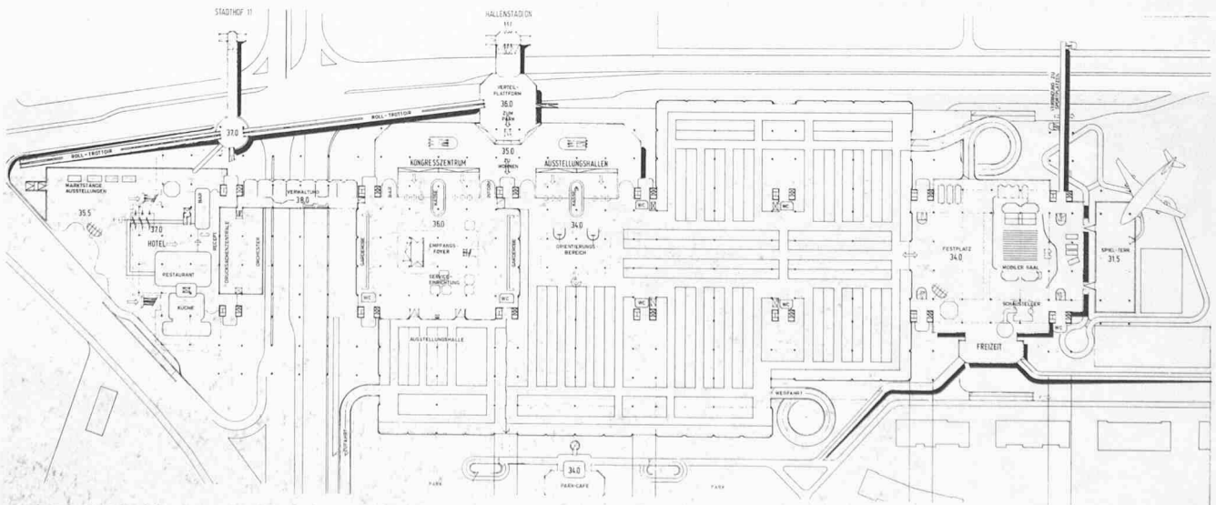
Eingangsgeschoss 1:3000 (Niveau 34,0/36,0)
