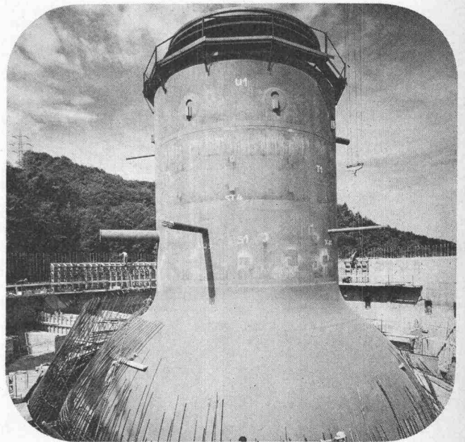
Wichtige Teile des Kernkraftwerks Mühleberg wurden mit Sécheron-Elektroden geschweisst.
