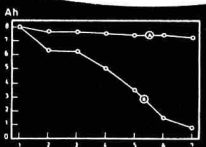
Fig. 10 Zyklusversuch mit antimonhaltigem (A) und antimonfreiem (B) Blei. Die Zyklen betragen aus wöchentlich einer Tiefentladung mit Kapazitätsbestimmung, die in dieser Figur aufgeteilt ist in tägliche Schwachentladungen nach J. Burban (7)
