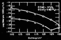
Fig. 14 Löslichkeitskurven und Antimonien in Schwefelsäure nach Ruetsch und Angstadt (7)
