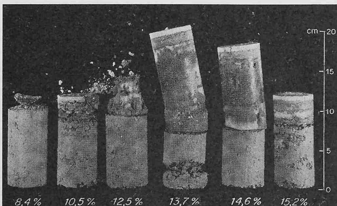
Bild 5. Frosthebungen eines kalkstabilisierten Bodens [ 4\% \text{Ca}(\text{OH})_2 ]; Frostversuch unmittelbar nach Verdichtung
