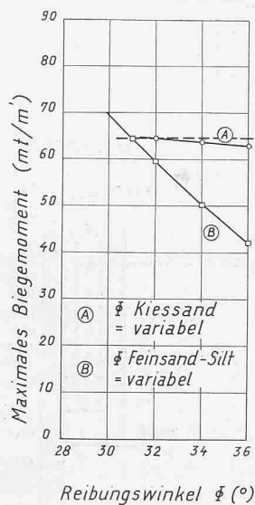
Einfluss der Scherfestigkeit auf das Moment
