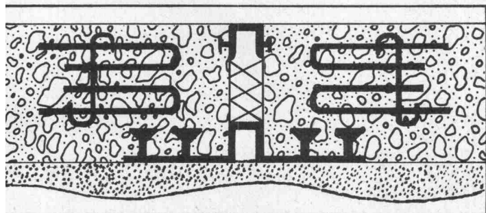
Reihe T/-Fugenband Oberflächenfugenbänder verhindern Eindringen von Grundwasser in die Betonfuge. Erhaltung der vollen Vand- und Bodenstärke an den Betonfugen. Niedrige Einbaukosten.
