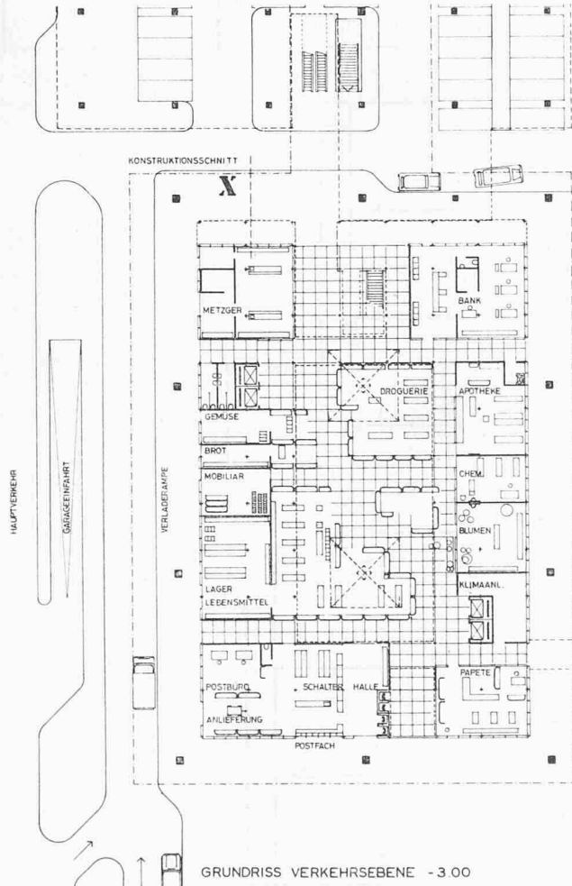
Zentrum 1:700, Verkehrsebene
