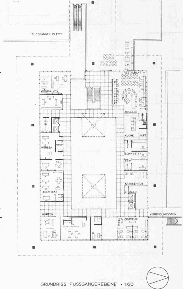
Fussgängerebene
