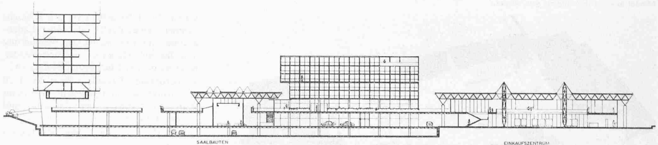
Zentrumsanlage, konstruktive Schnitte 1:200
