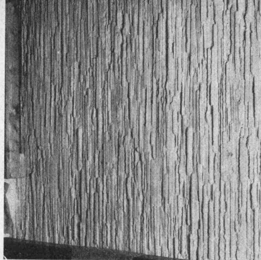
▲ Struktur «Pre-Dur» Vertikal-Innenraum Café-Motel, Chur. ◀ Struktur «Grave» Vertikal mit «Lecca»-Beton, Zoo Zürich, Elefantenhaus. Struktur «Grave» Horizontal, N 2-Autobahn Rothenburg LU. ▶
