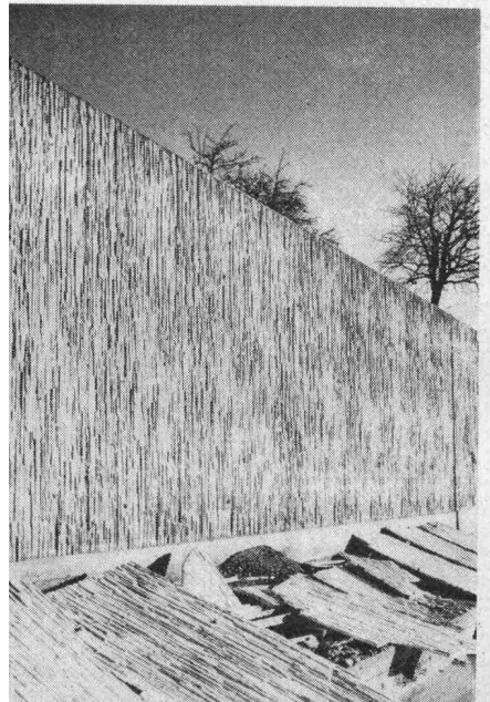
◀ Struktur «Pre-Dur» Vertikal, N 1-Autobahn Hagenbuch ZH. Struktur «Pre-Dur» Vertikal, Westtangente (14 000 m 2 ) Zürich. ▶ ▼ Struktur «Maestoso B», Balkonbrüstungen, Diessenhofen TG.
