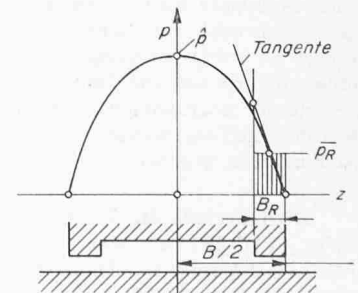
Bild 17.3. Näherungsberechnung der Druckverteilung in der Staurand-Zone
