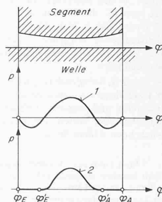
Bild 5.5 Druckverteilung im Fall b 3
