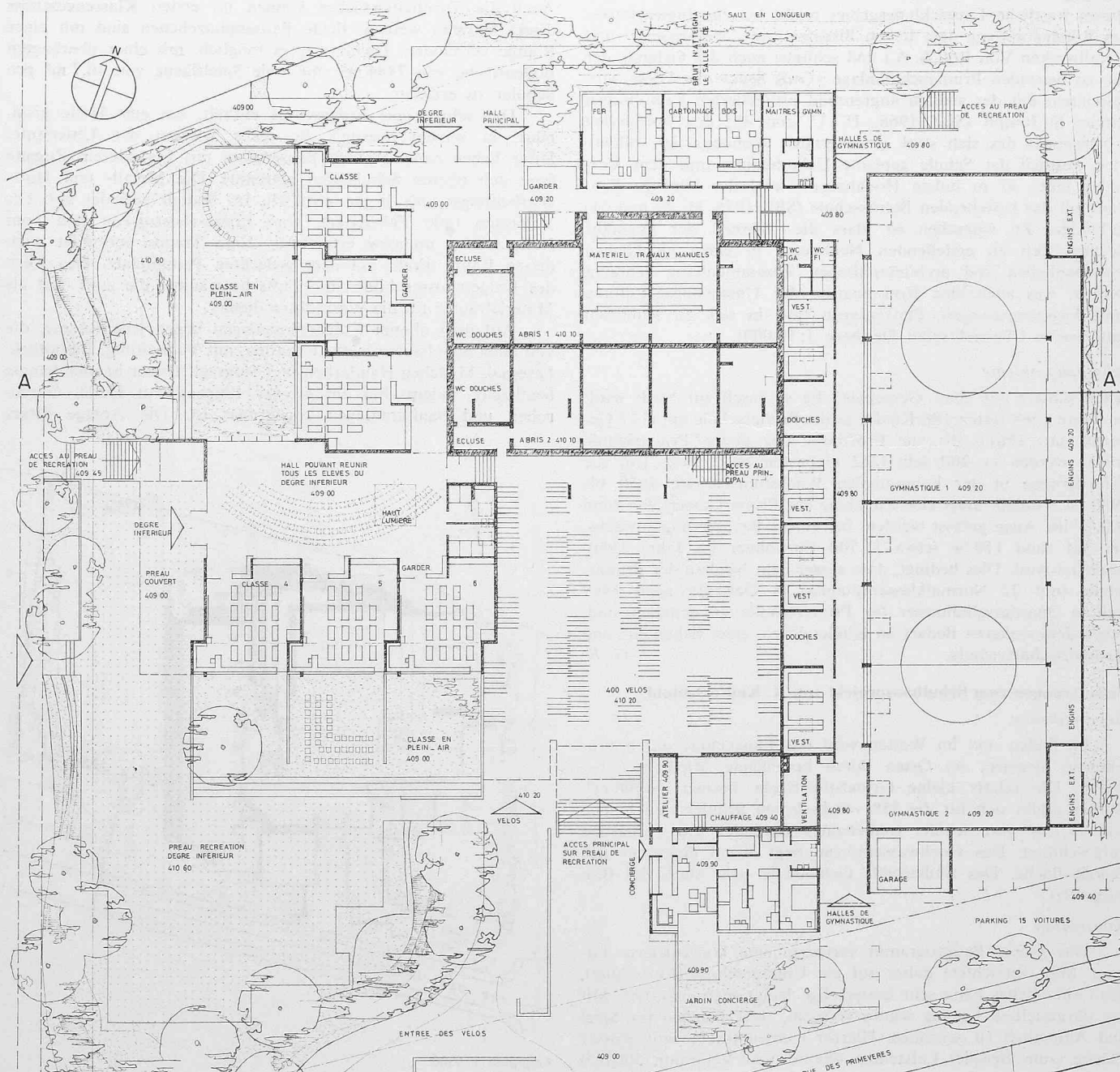
Unteres Eingangsgeschoss 1:500
