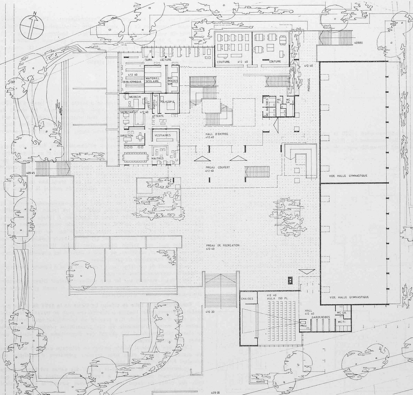
Oberes Eingangsgeschoss 1:500
