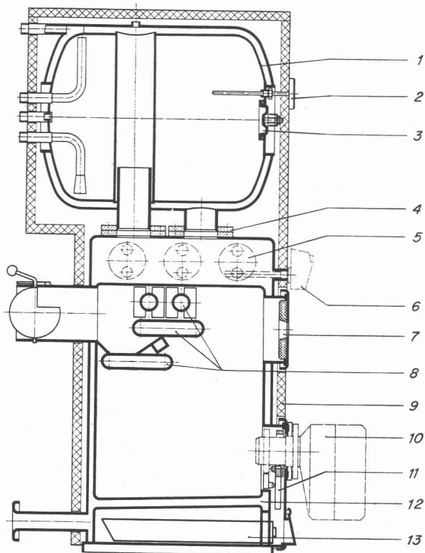
Bild 1. Schnitt durch den Idag-SB-Kessel
