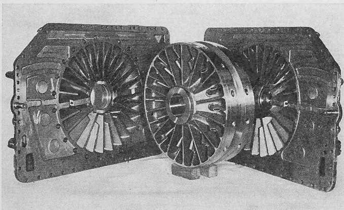
Bild 5. Beschauflte Teile (Rotor und Stator) einer doppelflutigen Voith-Strömungsbremse für Schienenfahrzeuge
