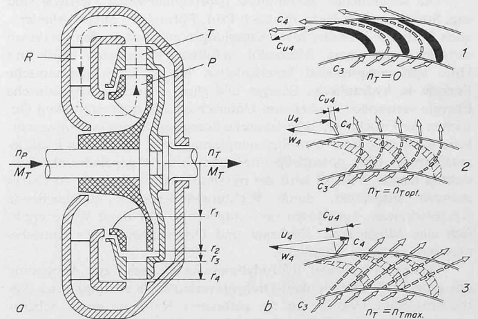
Bild 6. Einstufiger Föttinger-Wandler a Schematische Darstellung des Aufbaues b Schematische Darstellung der Strömung in der Turbinenbeschauflung bei den Betriebszuständen: 1 Stillstand, 2 bester Wirkungsgrad, 3 Durchgangsdrehzahl
