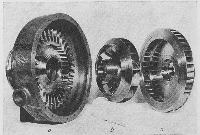
Bild 7. Beschauflte Teile eines Föttinger-Wandlers nach Bild 6 a Leitradgehäuse (a Reaktionsteil R), b Pumpenrad P, c Turbinenrad T
