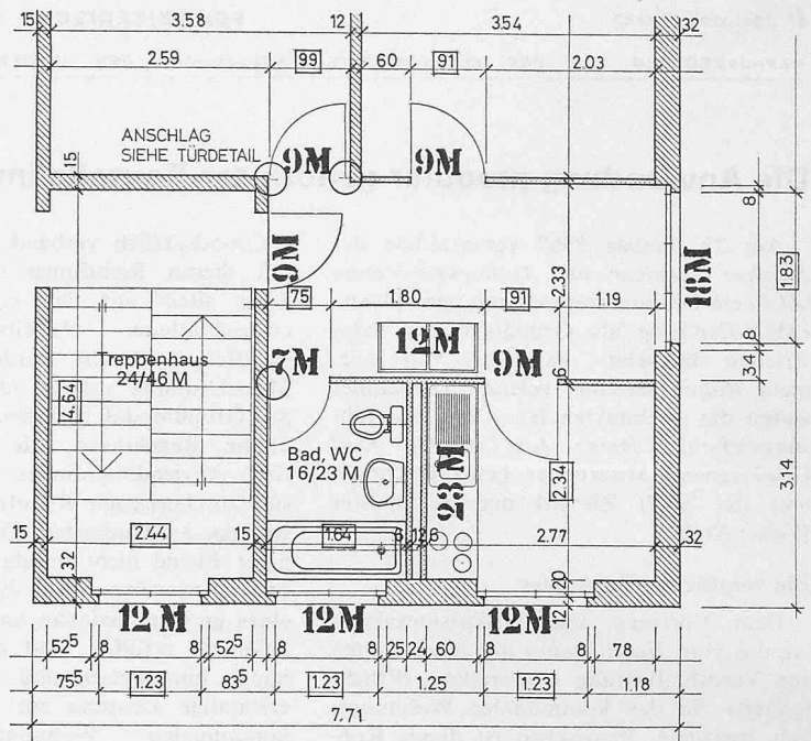
Bild 3. Ausführungsplan 1:100 eines modular vermassen Wohntypgrundrisses (vgl. Bild 2)
