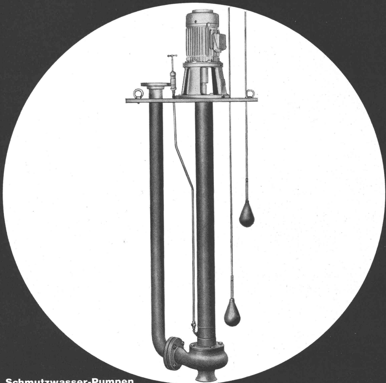
Schmutzwasser-Pumpen
