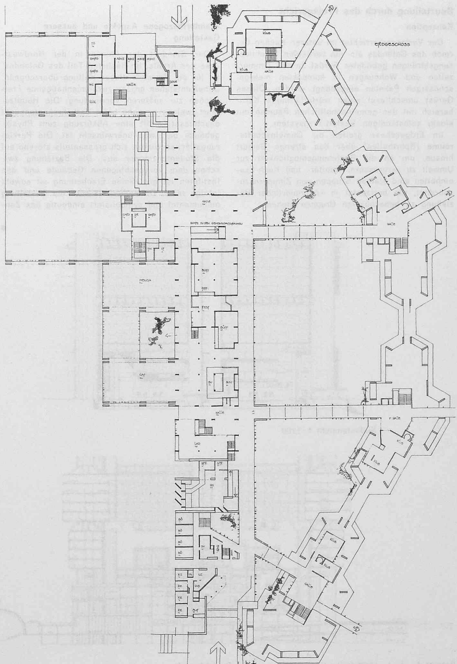
Obergeschoss 1:1200. Von unten nach oben im Komplex der Gemeinschaftsanlagen (links): Aufenthalt (Krankenstation), Ökumenisches Foyer (Luftraum), Musikzimmer, Ladenfläche, Freizeiträume, Bibliothek und Leseraum, Anschluss und Garderoben Schwimmhalle bzw. Turn-Sporthallen. Verbindungsstränge in die zentralen Hallen der vier Studentenhäuser (rechts)
