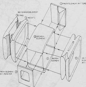
FRONTELEMENT MIT TÜR
