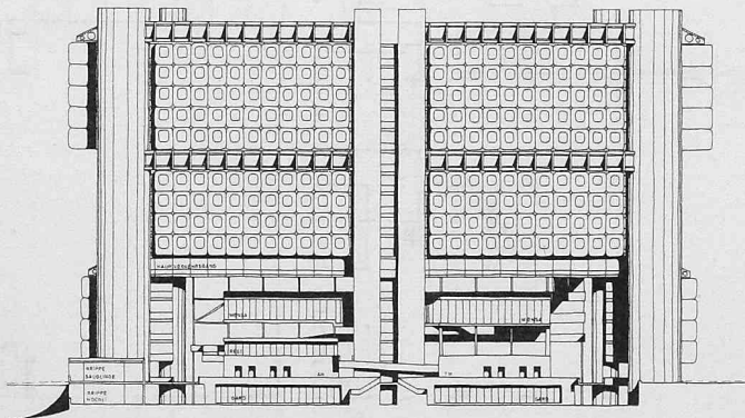
Südostansicht 1:1200
