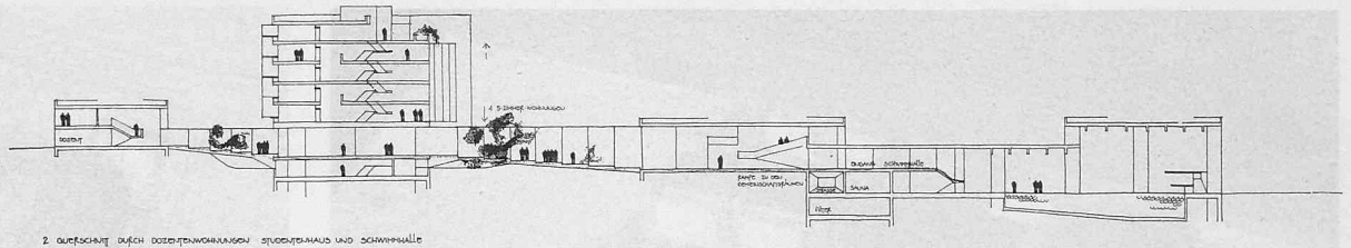
Querschnitt 1:1200. Von links (Osten) nach rechts (Westen): Dozentenwohnungen, Studentenhaus (mit vier Fünfstückerwohnungen), Verbindung zu den Sportanlagen (Schwimmhalle) und über Rampe zu den Gemeinschaftsräumen. Im Untergeschoss Verbindungsstrasse
