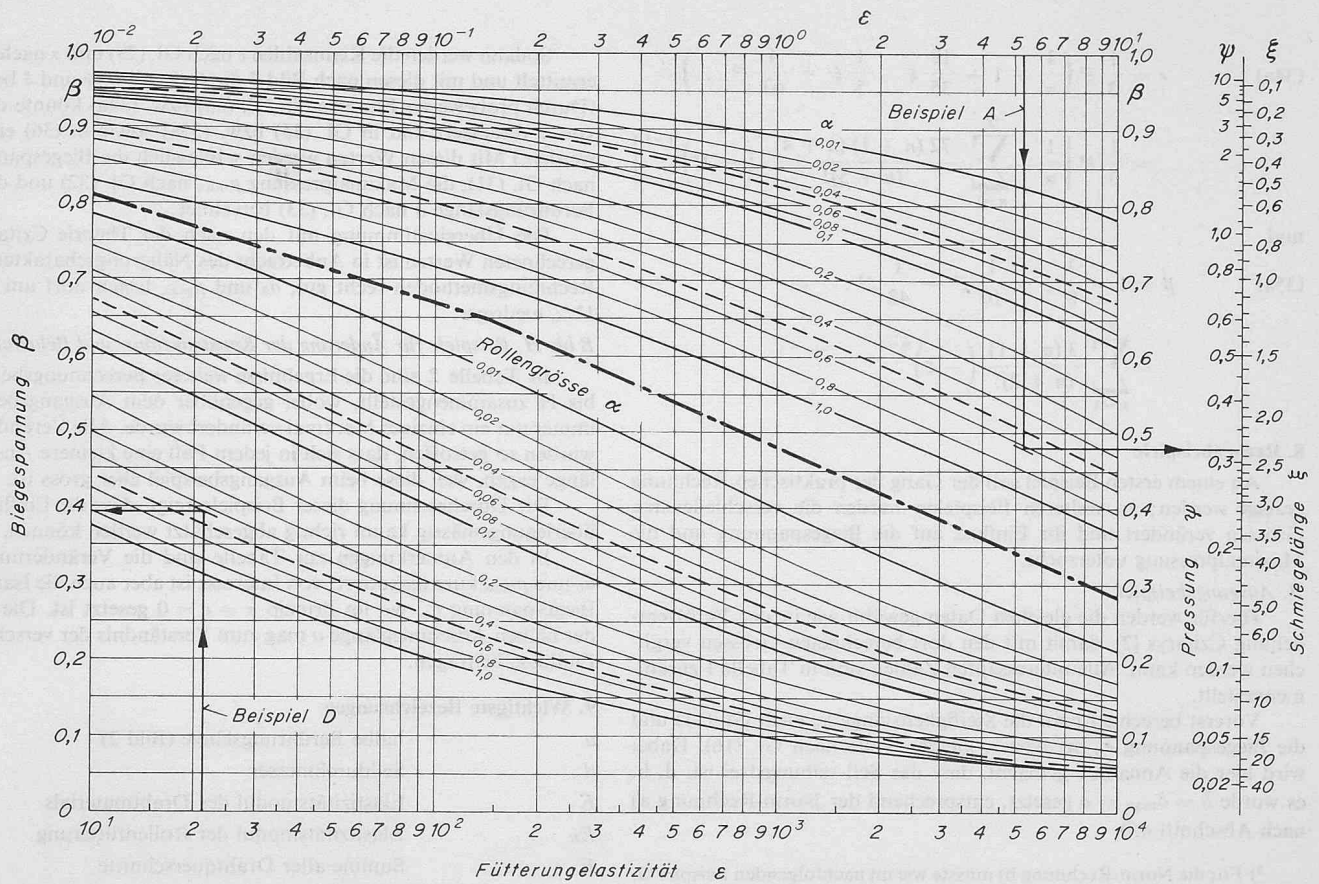
Bild 7. (Dimensionslose) Abhängigkeit der Biegespannung \beta und der Pressung \psi von der Fütterungselastizität \epsilon und der Rollengrösse \alpha ( \xi = Schmiegeleänge-Parameter)
