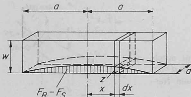
Bild 6. Gedrückter Teil der Rollenfütterung (rektifiziert und idealisiert: wirksame Fütterungsbreite = Seildurchmesser d ; wirksame Fütterungsdicke = w )
