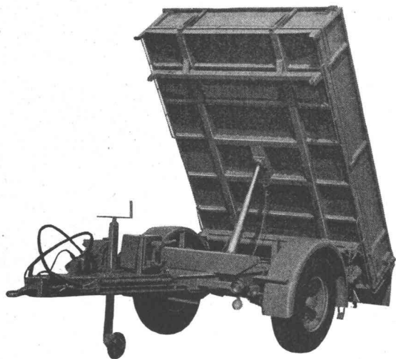
Dreiseitenkipper für Unimog, Jeep, Land-Rover usw.
