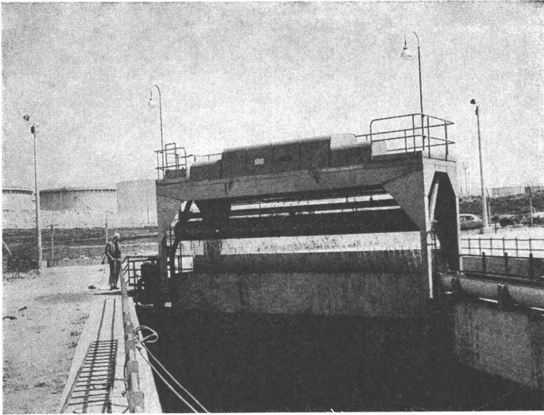
Rechen- und vollautomatische Rechenreinigungs-Maschine einer Petro raffinerie am Mittelmeer. Breite des Rechens und der Putzharke 8 m.
