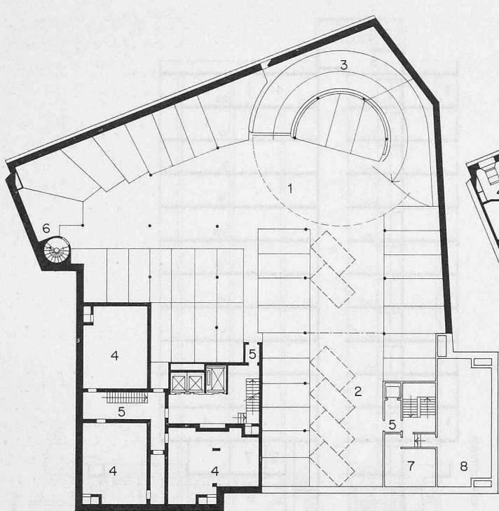
Zweites Untergeschoss 1:500
