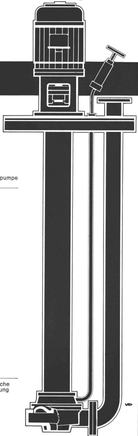
2 HÄNY-Normschacht
