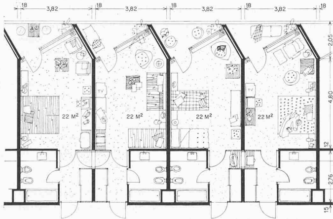
DOPPELZIMMER MIT LOGGIA (1-3. ZIMMERGESCHOSS)
