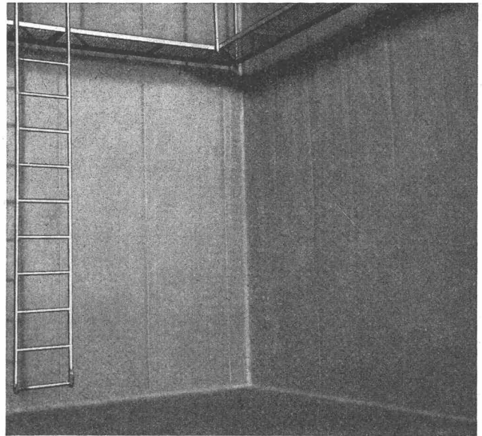
Innenauskleidung eines 250 000 I Betontankes Revêtement intérieur d'une citerne en béton de 250 000 I
