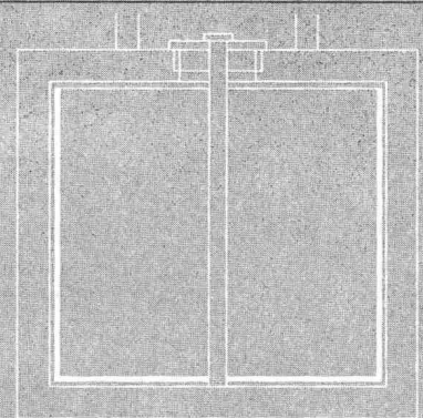
Innenauskleidung eines 250 000 I Betontankes Revêtement intérieur d'une citerne en béton de 250 000 I
