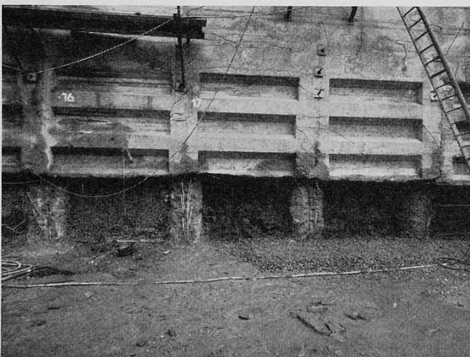
Bild 11. Neubau der TT-Direktion an der Wallstrasse in Basel: Aufgelöste Pfahlwand
