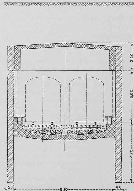
Bild 7. U-Bahn Mailand: Tunnelquerschnitt mit Pfählwand als Seitenabschluss
