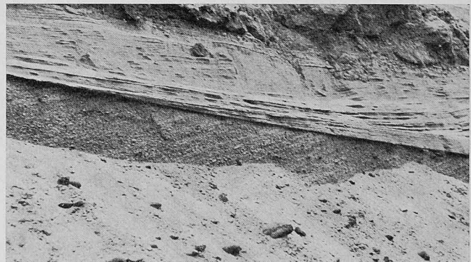
Bild 9. Lagerungsverhältnisse von sandig-kiesigen Ablagerungen in einem Geländeanschnitt
