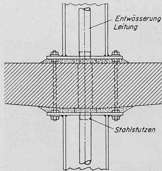
Bild 9b. Querschnitt durch die Verankerungsplatte/Stütze
