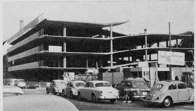
Bild 4. Ansicht des fertig montierten Parkhauses von der Stirnseite mit teilweise montiertem Gelände, Treppenhäuser noch nicht montiert
