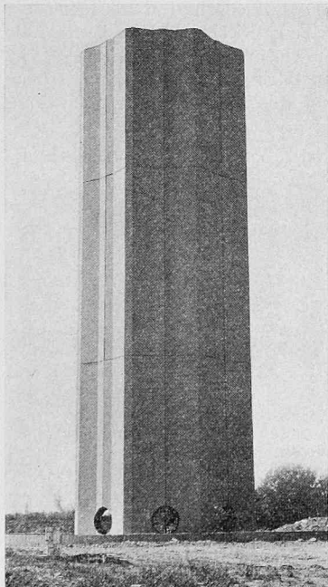
Bild 8. Kühlturm aus vorgespannten Falterkswänden
