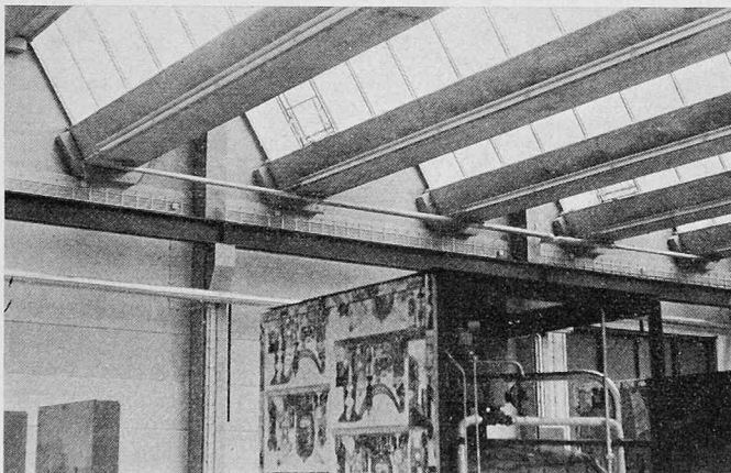
Bild 14. «Z»-Faltwerkshalle in Berlin für 15,0 m Spannweite. Arch.: Harry May, Berlin, Ausführung: Imbau, Deckbergen
