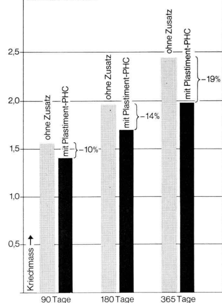
Kriechversuche
