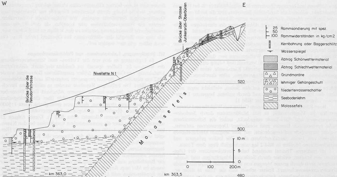
Bild 3. Beispiel eines typischen geotechnischen Längsenprofils für das Ausführungsprojekt der N 1, Abschnitt Oberbüren—St. Gallen, Gebiet nahe südlich Niederbüren, vereinfacht
