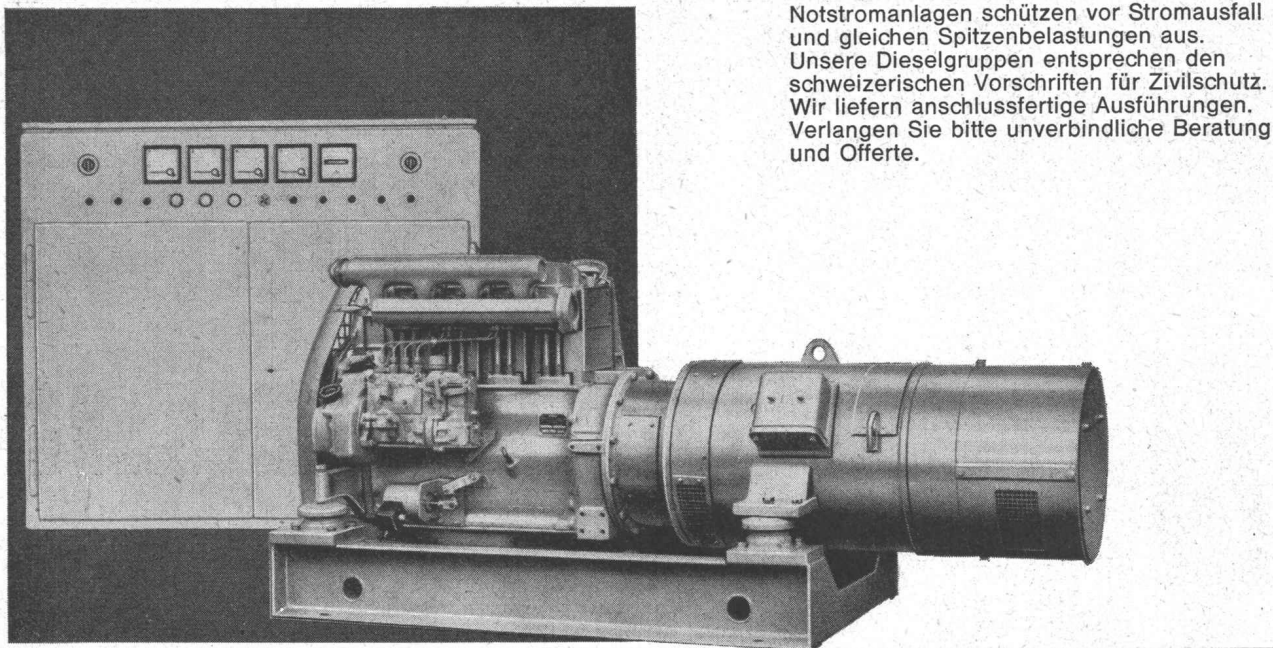
24 KVA, 3x380 V, 50 Hz, mit Dieselmotor Leistungsbereich: ab 600W, nach oben unbeschränkt
