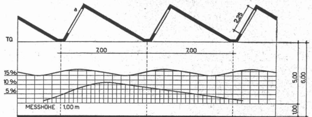
Scheddach mit schrägen Glasflächen Mittelwert 16,8%
