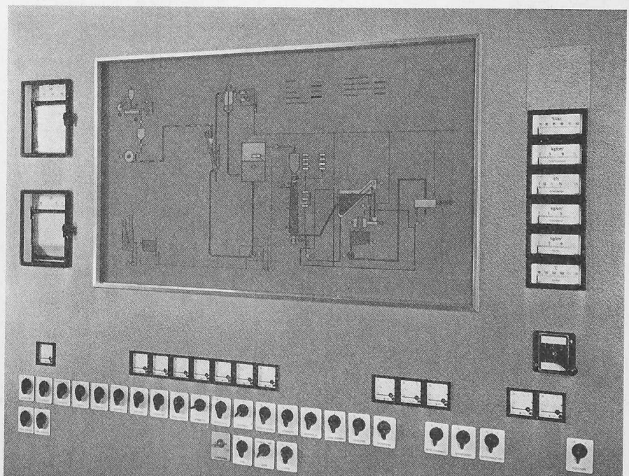
Bild 6. Schalt- und Steuerwarte für eine Escher Wyss-Halbzellstoff-Anlage mit Leuchtschaubild
