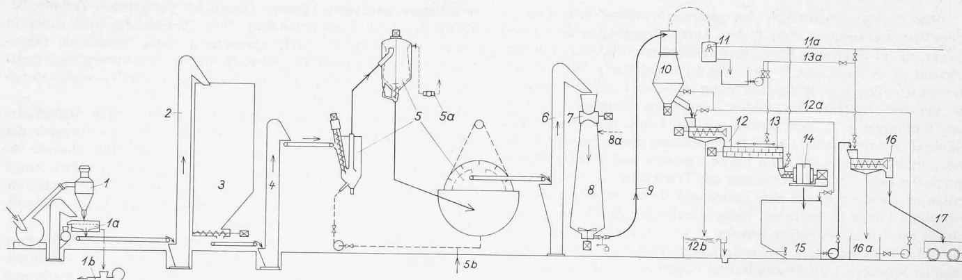
Bild 9. Fließschema einer Halbzellstofffabrik mit kontinuierlicher Escher Wyss-Anlage.
