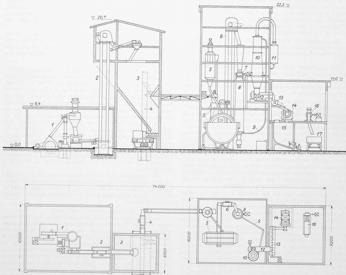
Bild 10. Aufstellungsplan der Anlage nach Bild 9.
