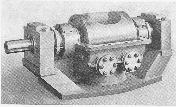
Bild 4. Escher Wyss-Drehventil (Typ DV 500 Z-25) zum Eintrag der getränkten Schnitzel in den unter Druck stehenden Kocher. Die obere Gehäusehälfte mit Verschleissbüchse ist entfernt. Das Bild zeigt Lagerbock und Rotor mit Stopfbüchsen zum Abdichten der Wellenenden.
