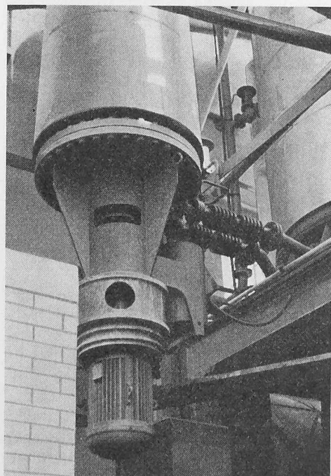
Bild 5. Kocherunterteil mit Antrieb für Schaufelrührer am Kocherboden und Ausblaseleitungen zum Blastank (Anlage Marsoni)
