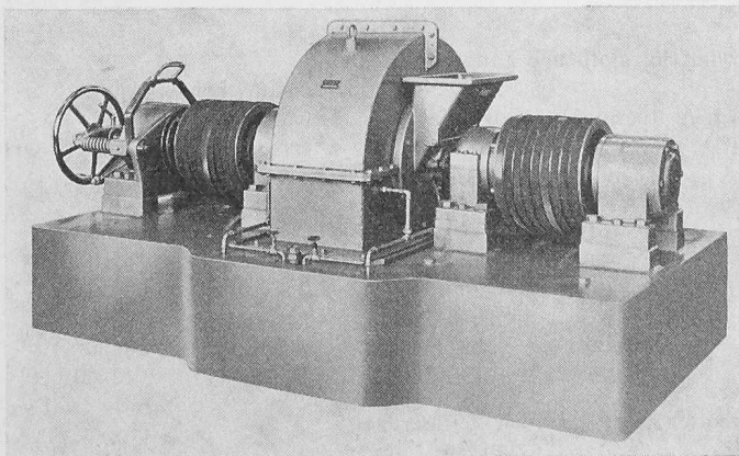
Bild 2. Escher Wyss-Doppelscheiben-Refiner zur Defibrierung (bzw. zum mechanischen Aufschluss) von Halbzellstoff. Die beiden unter dem Gehäusedeckel angeordneten und mit Mahlsegmenten versehenen Scheiben arbeiten gegenläufig. Stoffeintritt über Zuführtrichter rechts am Gehäusedeckel. Einstellung des Scheibenabstandes über Handrad und Spindel (links).
