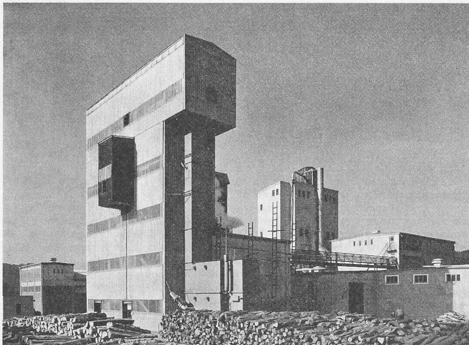
Bild 1. Kontinuierliche Escher Wyss-Halbzellstoffanlage bei der Firma Hamburger in Pitten/Niederösterreich Imprägnier-, Aufschluss- und Entspannungsteil der Anlage sind in der verkleideten Stahlkonstruktion untergebracht, aus der lediglich der Tränkbehälter (Bildmitte) herausragt. Die mechanische Stoffaufbereitung des Halbzellstoffes befindet sich im anschliessenden Gebäude.
