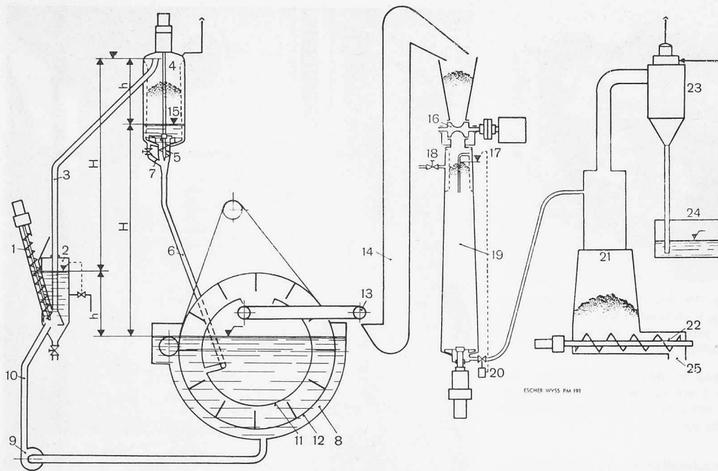
Bild 7. Schematische Darstellung des Escher Wyss-Prinzips zur kontinuierlichen Halbzellstoffherstellung.
