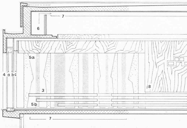
Ansicht der Aula-Rückwand mit Schnitt durch Saalfenster, 1:150
