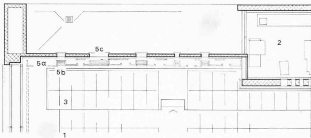
Grundriss der schallabsorbierenden Aula-Rückwand 1:150
