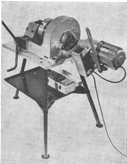
Gewindeschneideapparat GA 4 mit elektrischem OGA-Antrieb auf dem neuen +GF+ Apparateständer
