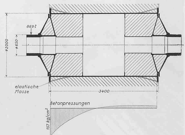
Bild 2 (rechts). Auflagetraverse, Schnitt 1:75 mit Verteilung der Betonpressungen
