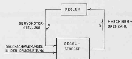
Bild 2 Der Regelkreis
